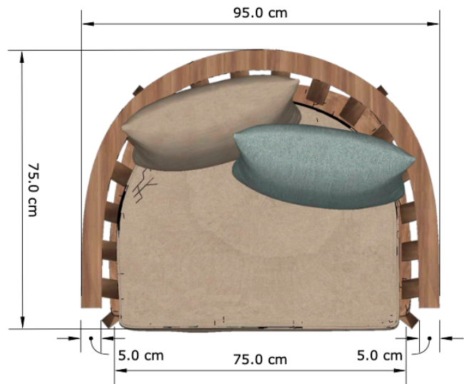
VISTA SUPERIOR
