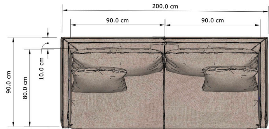
VISTA SUPERIOR
